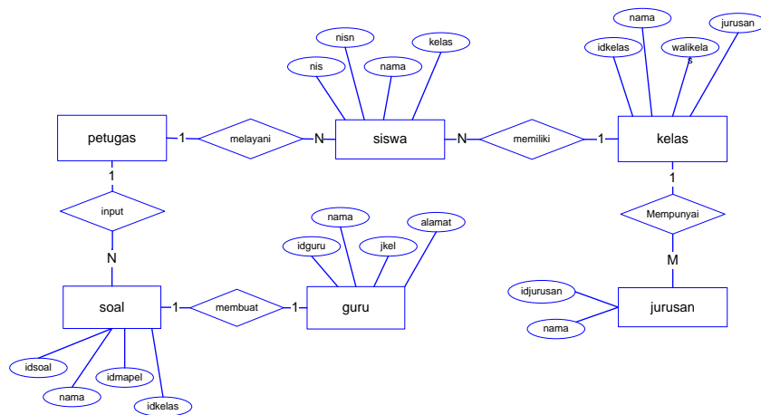
Gambar 4. ERD
