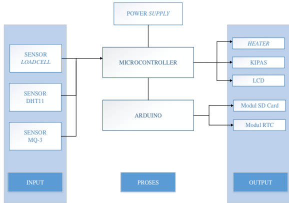
Gambar 4. perancangan Hardware
