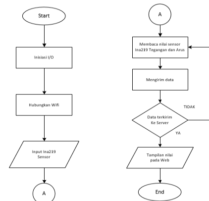
Gambar 3. Flowchart Pemrograman
