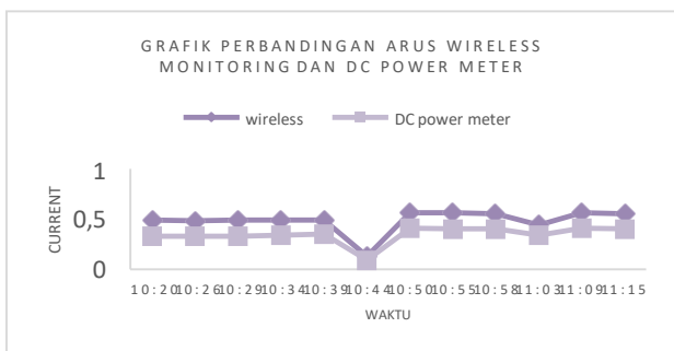
Gambar 10. Grafik Pengujian Arus Solar Cell
