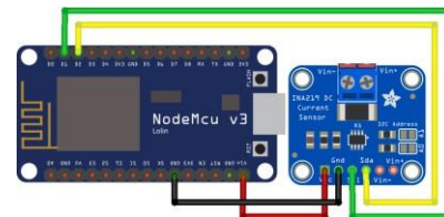
Gambar 2. Perancangan ESP8266 dan INA219
