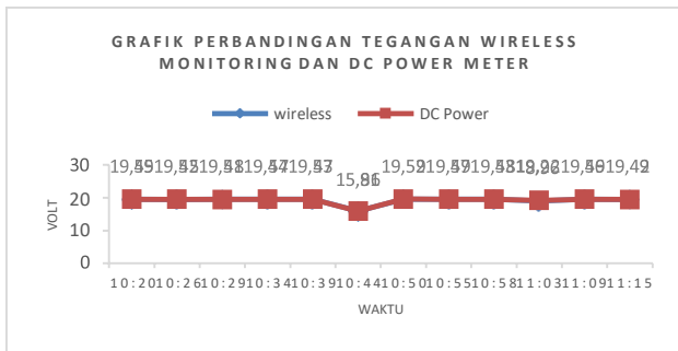
Gambar 9. Grafik Pengujian Tegangan Solar Cell
