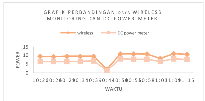
Gambar 11. Grafik Pengujian Daya Solar Cell
