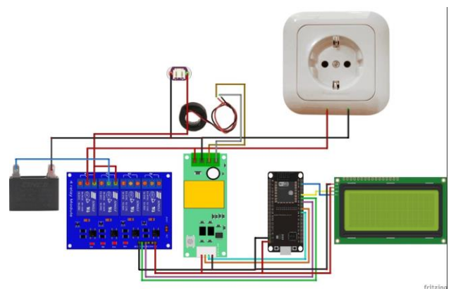
Gambar 2. Desain Kabel
