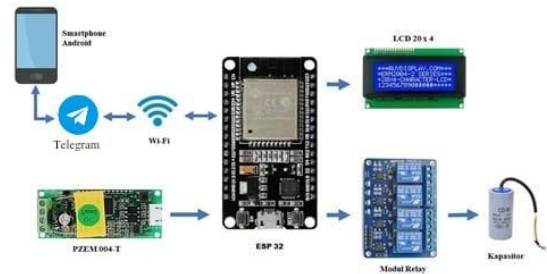
Gambar 1. Desain Sistem
