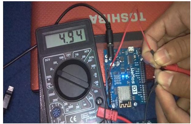
Gambar 9. Pengukuran Tegangan Pin Output 5v Arduino Wemos D1
