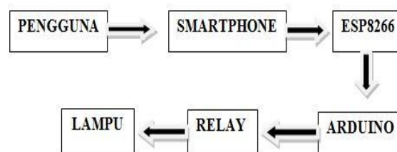
Gambar 1. Diagram Blok Desain Alat Pengoperasian Lampu Dengan Esp8266 Melalui Web Browser Aplikasi Android Berbasis Mikrokontroler
